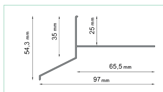
PROFIL OKAPOWY D25
