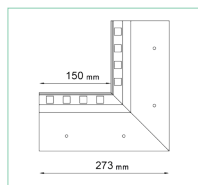
NAROŻNIK WEWNĘTRZNY W30 90
