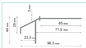
PROFIL OKAPOWY K100R
