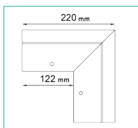
NAROŻNIK ZEWNĘTRZNY K100R 90
