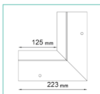
NAROŻNIK WEWNĘTRZNY K100R 90
