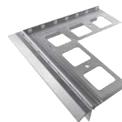
Narożnik zewnętrzny K20R 90°
