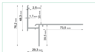
PROFIL OKAPOWY W35 PLUS
