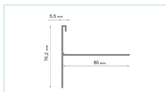
PROFIL OKAPOWY BOCZNY W35B
