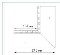
NAROŻNIK WEWNĘTRZNY W35 PLUS 90
