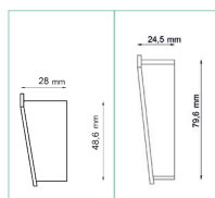
ODBOJNIKI PRZYŚCIENNE P+L OPW20/ OPW20R/ OPW35 PLUS
