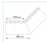
NAROŻNIK WEWNĘTRZNY W35 PLUS 135
