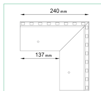
NAROŻNIK ZEWNĘTRZNY W35 PLUS 90
