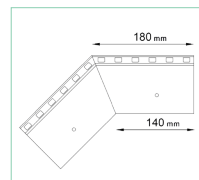
NAROŻNIK ZEWNĘTRZNY W35 PLUS 135
