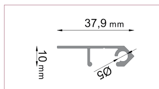
PROFIL COKOŁOWY C LED
